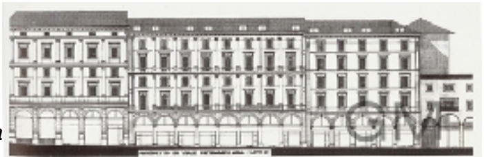
Prospetto su viale Pietramellara
